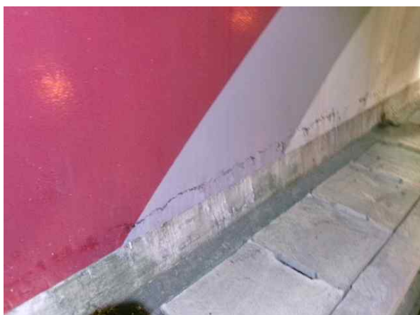
라이닝 S28 측벽부 균열( Cw=0.3\text{mm} 미만)-문산방향
